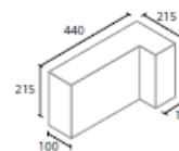
L-Block
